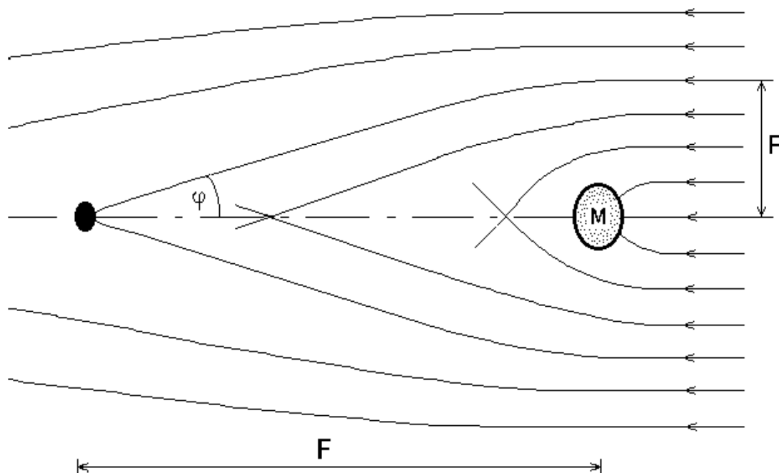
Рис.3. Фокусировка неподвижным гравитирующим объектом. Проходящий со скоростью v на расстоянии от центра объекта p=(2GMv)^{1/2} поток агента "схлопывается" в точке наблюдения. Наблюдатель воспринимает приходящий поток как кольцо с угловым радиусом \varphi \approx p/F .
