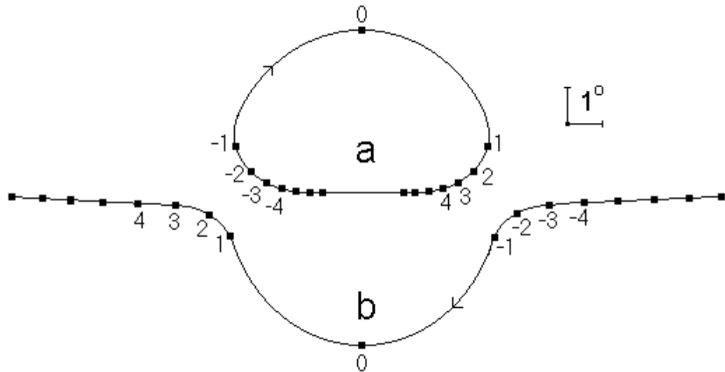
Рис.4. Влияние Солнца на наблюдаемое положение относительно звезд источника потока частиц, имеющих скорость 500 км/с, при тесном угловом сближении неотклоненного положения с центром Солнца (минимальное расстояние - 12 угловых минут) [13]. Цифрами обозначены наблюдаемые положения источника с интервалом в 1 сутки; нулю соответствует минимальное угловое расстояние между центром Солнца и неотклоненным направлением на источник; a - первичный "источник", b - возникающий и исчезающий "источник".
