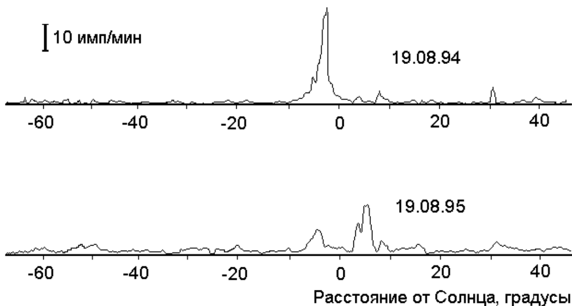
Рис.6. Всплески сигнала во время сближения центра Солнца со звездой \eta Льва (минимальное расстояние 5 угловых минут). Телескоп: стальное параболическое зеркало с фокусным расстоянием 10 см, детектор - счетчик Гейгера диаметром 2 мм и длиной 6 мм [8].
