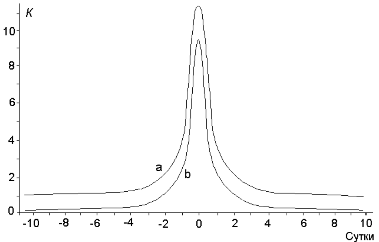
Рис.5. Расчетное изменение плотности потока проходящих вблизи Солнца мононаправленных частиц, имеющих скорость 500 км/с, при угловом сближении направления потока и направления на центр Солнца (минимальное расстояние - 12 угловых минут) [13]. По горизонтальной оси - время от момента наиболее тесного сближения; a - первичный "источник", b - возникающий и исчезающий "источник".
